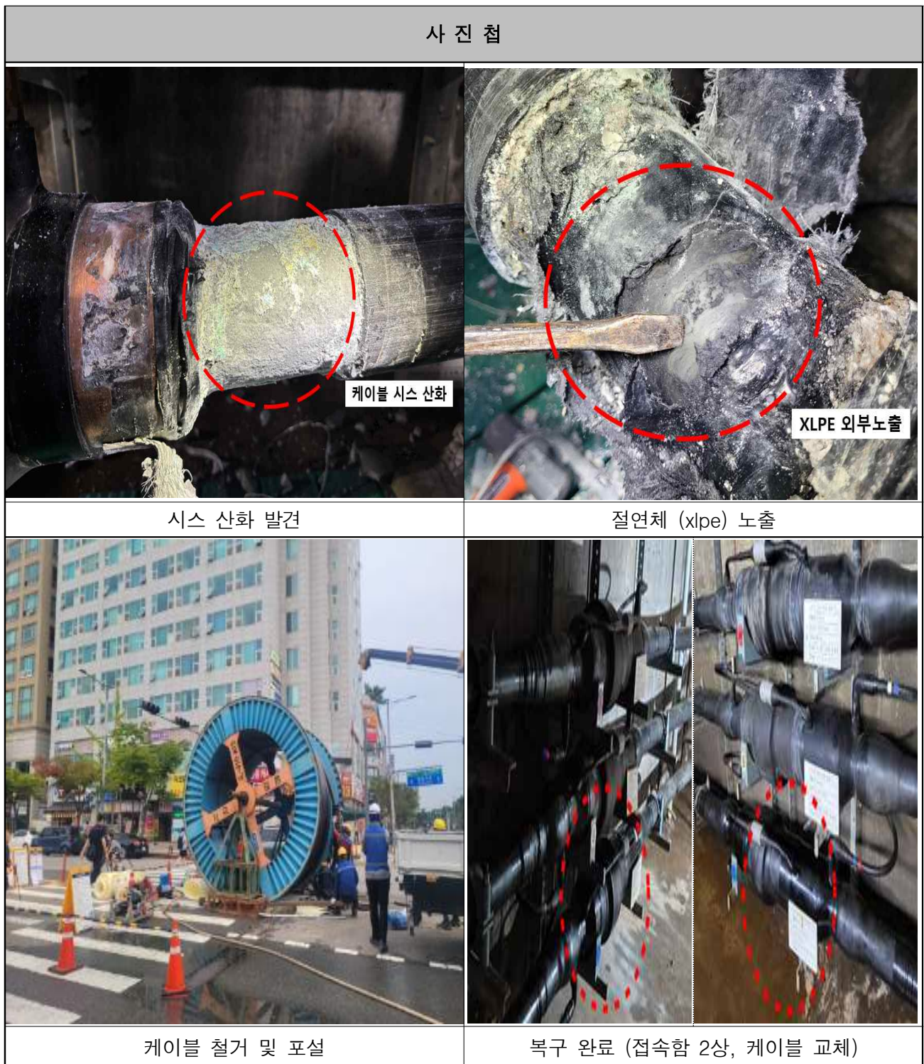
[그림 4] 154kV 영종-을왕 T/L 수분침투 긴급 복구공사 사진
